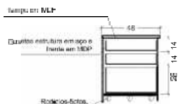
Figura 74 Corte | Escala 1:50
