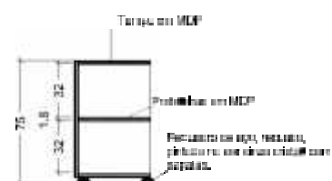
Figura 68 Corte | Escala 1:50
