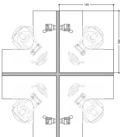
Figura 05 Estação de Trabalho ETA 4 - 160X140X60cm Vista superior | Escala 1:50
