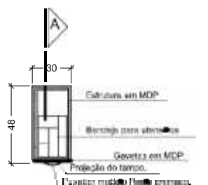
Figura 75 Visa superior | Escala 1:50
