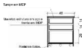
Figura 77 Corte | Escala 1:50
