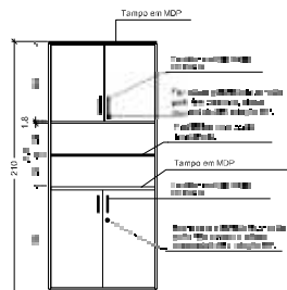
Figura 61 Elevação | Escala 1:50
