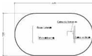
Figura 25 Mesa de retangular (tampo único com calha e calha de tomadas) MRRt 4 - 220x120cm Vista superior | Escala 1:50
