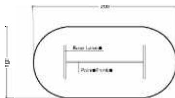
Figura 22 Mesa retangular (tampo único) MRRt 1 - 200X100cm Vista superior | Escala 1:50
