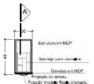
Figura 72 Visa superior | Escala 1:50
