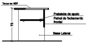
Figura 34 Corte | Escala 1:50
