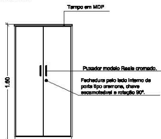
Figura 51 Elevação | Escala 1:50
