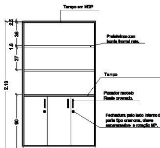
Figura 63 Elevação | Escala 1:50
