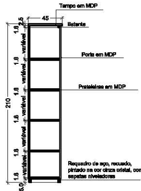
Figura 55 Corte | Escala 1:50
