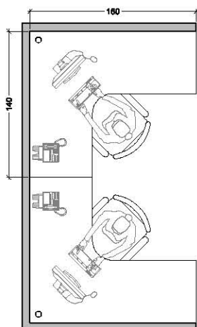
Figura 05 Estação de Trabalho ETA 2U-A - 160X140X60cm Vista superior | Escala 1:50
