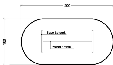
Figura 27 Mesa retangular (tampo único) MRRt 1 - 200X100cm Vista superior | Escala 1:50
