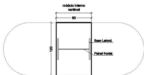
Figura 32 Mesa de retangular (tampo interno retangular) MRRt 8 - 80x120cm Vista superior | Escala 1:50
