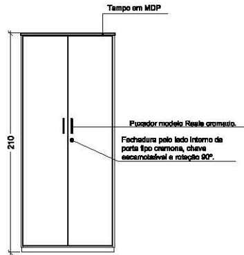
Figura 54 Elevação | Escala 1:50
