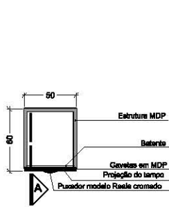
Figura 56 Vista superior | Escala 1:50
