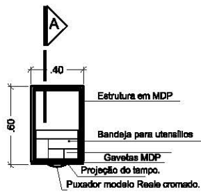
Figura 74 Vista superior | Escala 1:50
