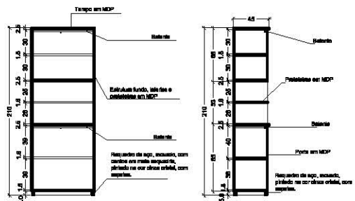
Figura 61 Cortes | Escala 1:50
