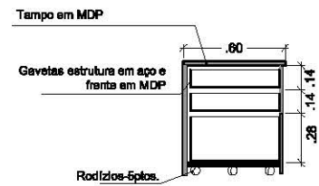
Figura 76 Corte | Escala 1:50
