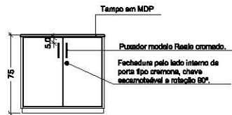
Figura 45 Elevação | Escala 1:50
