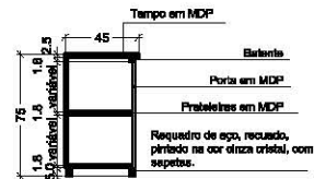
Figura 46 Corte | Escala 1:50
