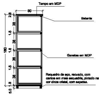
Figura 58 Corte | Escala 1:50
