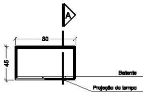
Figura 44 Vista superior | Escala 1:50
