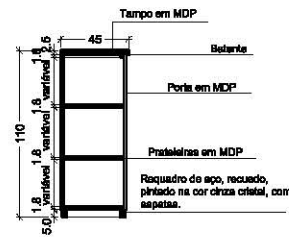
Figura 49 Corte | Escala 1:50
