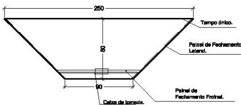
Figura 36 Mesa componível Trapezoidal (com calha na largura menor) MCT 1 - 80x250x90cm Vista superior | Escala 1:50
