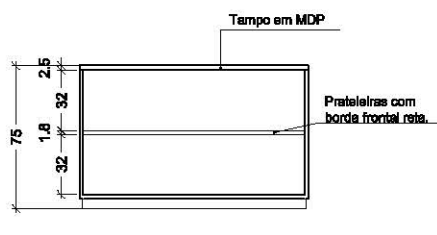
Figura 66 Elevação | Escala 1:50
