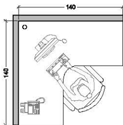
Figura 08 Estação de Trabalho ETB 1 - 140X140X60cm Vista superior | Escala 1:50
