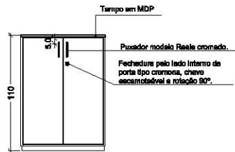
Figura 48 Elevação | Escala 1:50
