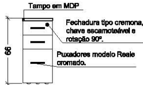
Figura 72 Elevação | Escala 1:50
