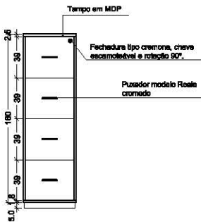
Figura 57 Elevação | Escala 1:50
