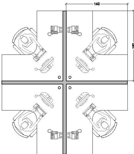
Figura 07 Estação de Trabalho ETA 4 - 160X140X60cm Vista superior | Escala 1:50
