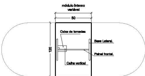
Figura 33 Mesa de Reunião Retangular (tampo interno retangular com calha e caixa de tomada) MRRt 9 - 80x120cm Vista superior | Escala 1:50
