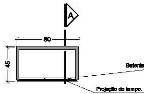
Figura 47 Vista superior | Escala 1:50
