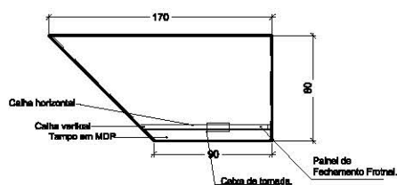
Figura 38 Mesa componível Trapezoidal (para fechamento) MCT 3 - 80x170x90cm Vista superior | Escala 1:50
