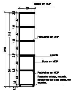
Figura 64 Corte | Escala 1:50
