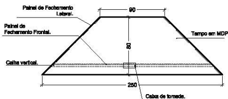
Figura 37 Mesa componível Trapezoidal (com calha na largura maior) MCT 2 - 80x250x90cm Vista superior | Escala 1:50
