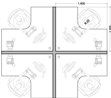
Figura 17 Estação de Trabalho ETC 4 - 140x120x60cm Vista superior | Escala 1:50
