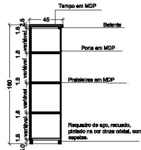
Figura 52 Corte | Escala 1:50
