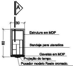
Figura 71 Vista superior | Escala 1:50
