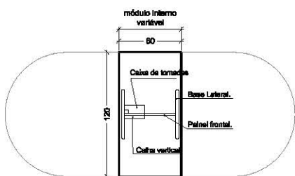
Figura 31 Mesa de retangular (tampo interno retangular com calha e caixa de tomada) MRRt 7 - 60x120cm Vista superior | Escala 1:50
