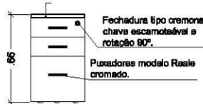
Figura 75 Elevação | Escala 1:50
