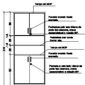
Figura 60 Elevação | Escala 1:50
