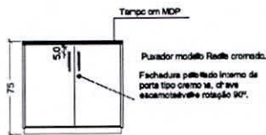
Figura 46 Elevação | Escala 1:50
