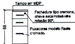
Figura 73 Elevação | Escala 1:50
