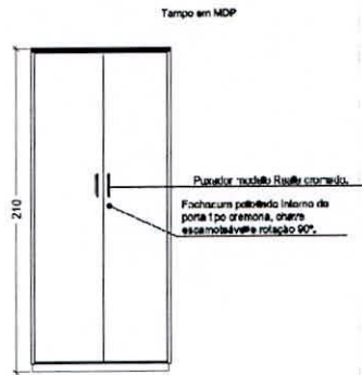
Figura 55 Elevação | Escala 1:50
