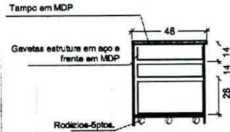
Figura 74 Corte | Escala 1:50
