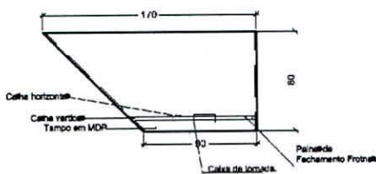
Figura 35 Mesa componível Trapezoidal (para fechamento) MCT 3 - 80x170x90cm Vista superior | Escala 1:50
