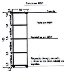
Figura 53 Corte | Escala 1:50
