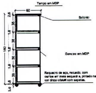
Figura 59 Corte | Escala 1:50
