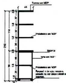
Figura 65 Corte | Escala 1:50
