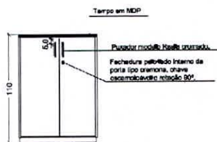
Figura 49 Elevação | Escala 1:50
