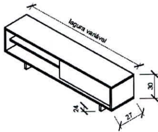
Figura 40 Nicho suspenso
