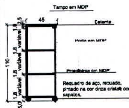
Figura 50 Corte | Escala 1:50
