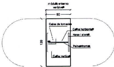
Figura 28 Mesa de retangular (tampo Interno retangular com calha e caixa de tomada) MRRt 7 - 60x120cm Vista superior | Escala 1:50
