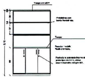
Figura 64 Elevação | Escala 1:50
