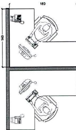
Figura 04 Estação de Trabalho ETA 2T-B - 160X140X60cm Vista superior | Escala 1:50
