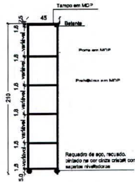
Figura 56 Corte | Escala 1:50
