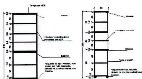
Figura 62 Cortes | Escala 1:50
