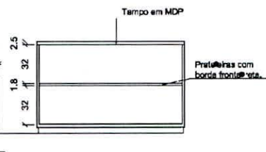
Figura 70 Elevação | Escala 1:50
