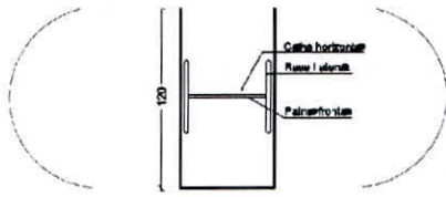
PLANTA SUPERIOR - MESA DE REUNIÃO RETANGULAR - MRRt 6 ESCALA 1:25
